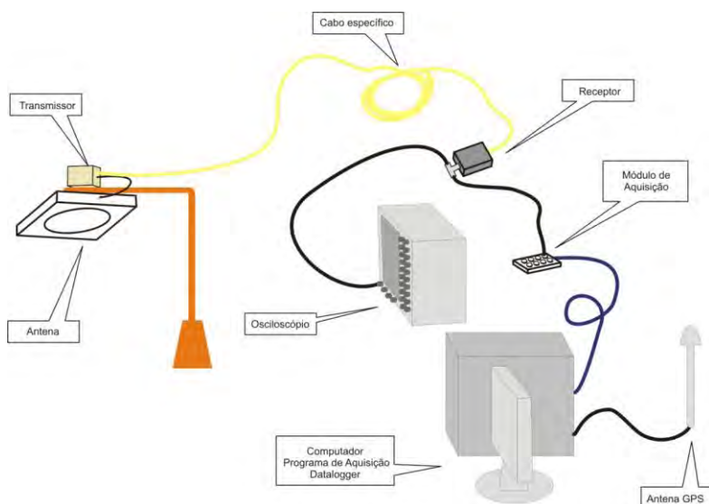
Figura 2.8 Esquema de montagem do campo elétrico lento
