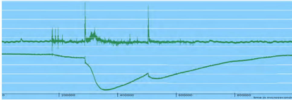
Figura 2.9 Exemplo de forma de onda de campo elétrico rápido (acima) e lento (abaixo) de um raio positivo da base de dados deste trabalho.
