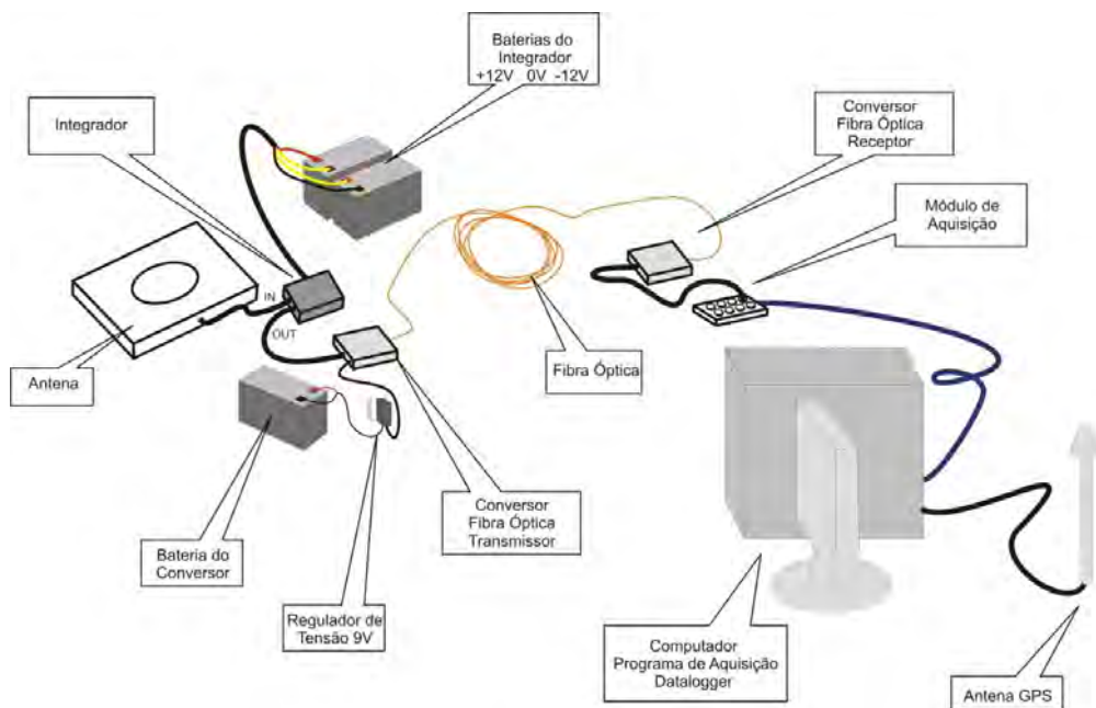
Figura 2.7 Esquema de montagem do campo elétrico rápido
