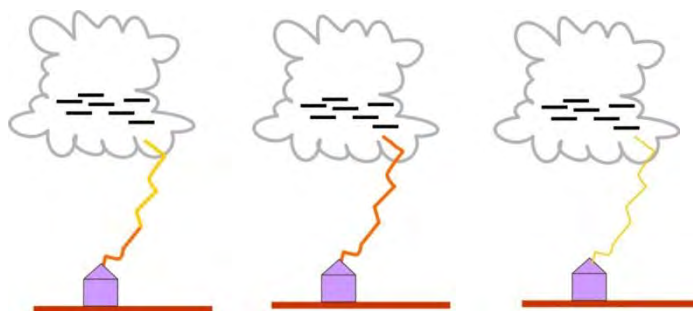
Figura 1.8 (a) Descarga conectante no momento que conecta ao líder (b) Descarga de retorno (c) transferência de carga contínua
