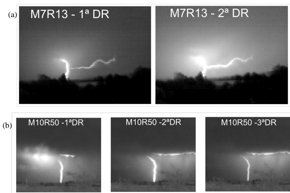
Figura 3.25 - Imagens das câmeras de alta velocidade dos casos de bipolares que utilizam o mesmo canal.
