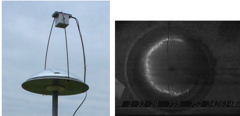
Figura 2.10 (a) Câmera e espelho usado na gravação de imagens da câmera allsky (b) Raio positivo registrado pela allsky. A sua grande extensão horizontal exemplifica a dificuldade que as câmeras normais têm de filmar a descarga completa.
