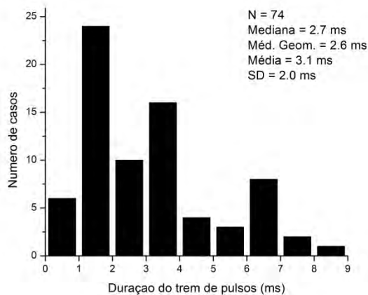
Figura 3.19 - Histograma da duração do trem de pulsos
