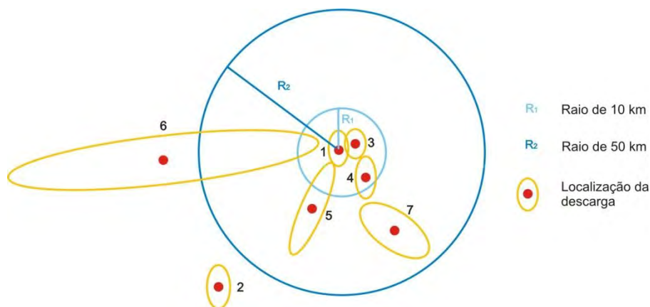
Figura 2.6 As descargas 1, 3, 4 e 5 serão associadas a um relâmpago enquanto as descargas 2, 6 e 7 serão atribuídas a outros relâmpagos
