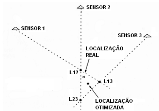
Figura 2.4 Localização do ponto de contato de uma descarga de retorno com o solo através do método da direção magnética, utilizando-se 3 sensores. L12, L13 e L23 são as intersecções das direções indicadas pelos sensores.
