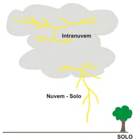
Figura 1.4 Classificação dos relâmpagos em função dos locais de origem e término
