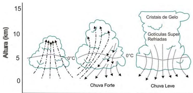
Figura 1.1 Representação dos estágios do ciclo de vida de uma nuvem cúmulo-nimbo
