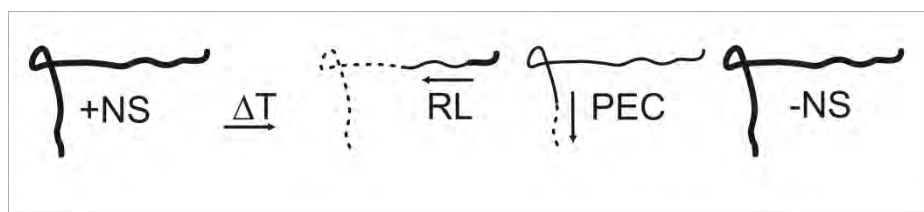
Figura 3.27 Esquemático da hipótese de raios bipolares que usam o mesmo canal
