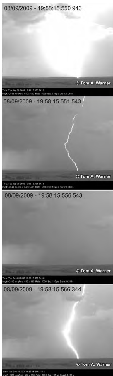
Figura 3.3 exemplo de raio múltiplo que utilizou o mesmo canal para se conectar ao solo.
