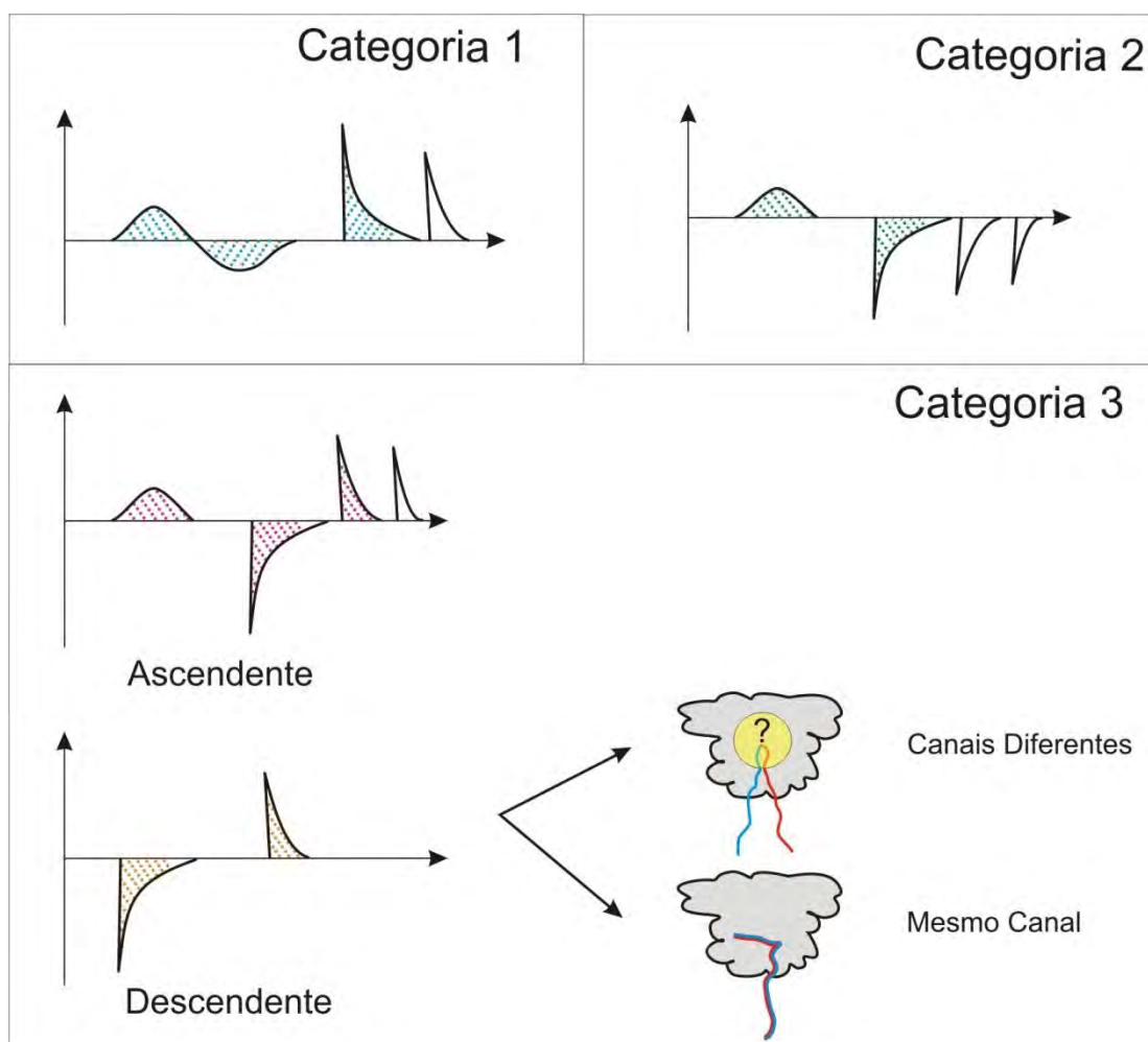
Figura 3.24 - Categorias de Bipolares encontrados na literatura.
