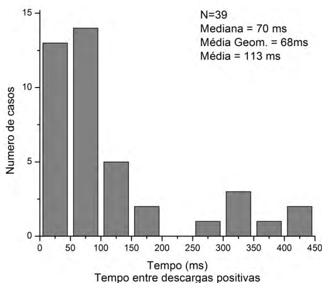
Figura 3.5 Distribuição do tempo entre descargas positivas
