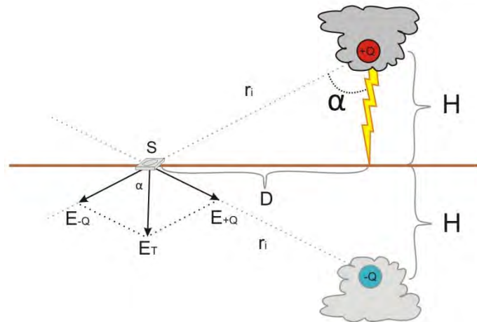
Figura 3.10 Representação gráfica do campo eletrostático que se desenvolve sobre o sensor, devido a uma carga espacial transferida +Q.
