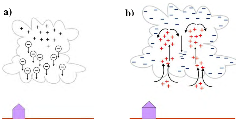
Figura 1.3 (a) Representação do transporte de cargas segundo a teoria gravitacional (b) Representação do transporte de cargas segundo a teoria convectiva.
