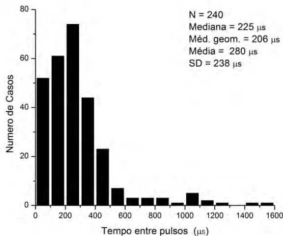
Figura 3.20 - Histograma do intervalo de tempo entre pulsos no trem de pulsos
